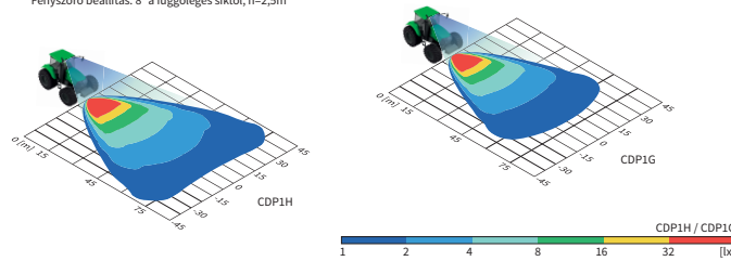
Az 1 lx fényintenzitás lehetővé teszi az újság olvasását Fényező beállítás: 8° a függőleges síktól, h=2,5m
