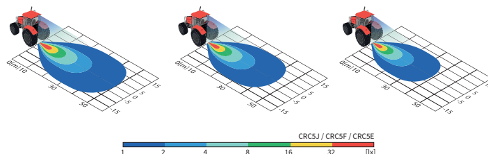
Fényszóró beállítás: 8° a függőleges siktól, h=2,5m
