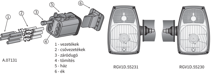
Deutsch DT 6-pin csatlakozó (opcionális)
