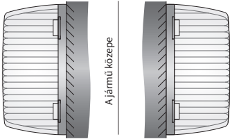
A lámpák elhelyezése a járművön (jármű előlnézete)
