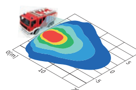
Az 1 lx fényintenzitás lehetővé teszi az újság olvasását Fényezőré beállítás: h=2,5m
